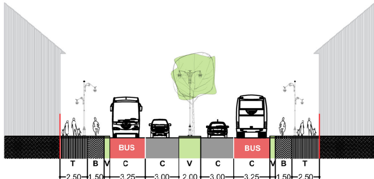
PROFIL STRADAL Str. Ștefan cel Mare
