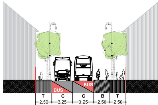
PROFIL STRADAL ex. Str. Piața Bernardy György, str. Mihai Viteazul
