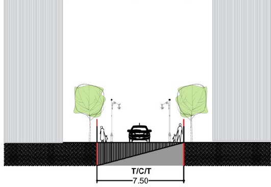
PROFIL STRADAL Străzi tip shared-space Ex. Str. Bolyai, Str. Târgului
