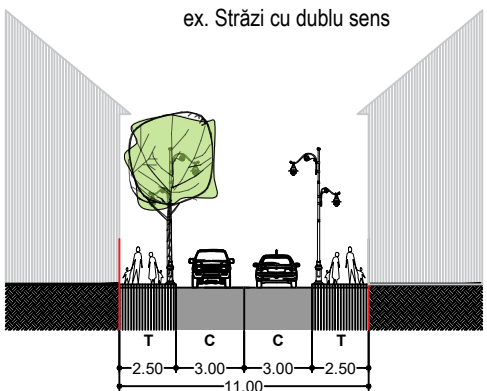
PROFIL STRADAL ex. Străzi cu dublu sens
