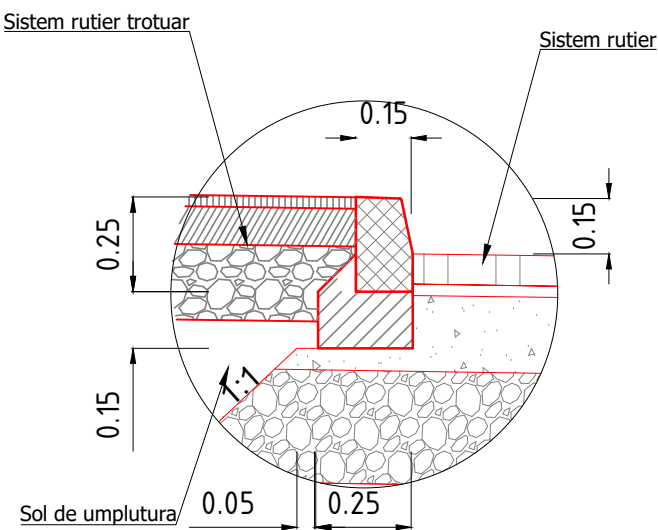
Nodul "A" - scara 1:20 -
